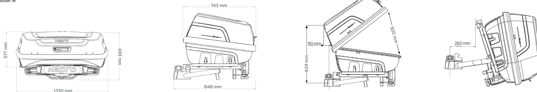
Afmetingen Boxer M
